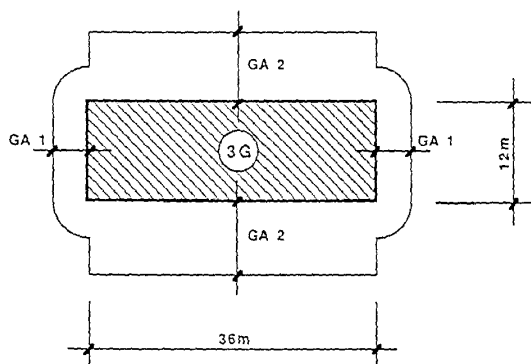
Abb. 1: einfache Baukörper
