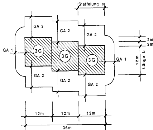
Abb. 2: lagemässig gestaffelte Baukörper
